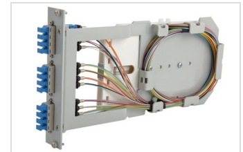
URM-Spleißmodul Seite 1
