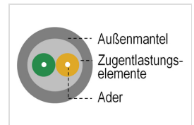
Uniboot-Duplexpatchkabel Querschnitt
