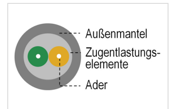
Uniboot-Duplexpatchkabel Querschnitt
