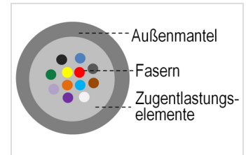
MPO Fanout-Kabel, Querschnitt
