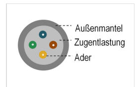
Minibreakoutkabel, Querschnitt
