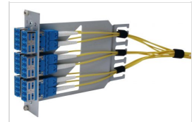
LWL-Patchmodul bestückt
