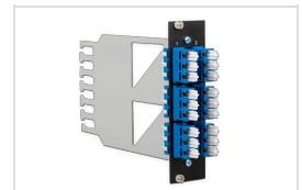
LWL-Patchmodul mit CS 3-port Kupplungen
