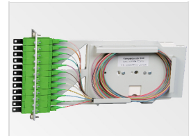
Kompaktspleißmodul
