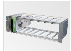
Kompaktspleißmodul im 3 HE Baugruppenträger
