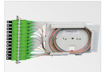
Kompaktspleißmodul
