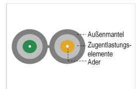
Duplexpatchkabel Querschnitt
