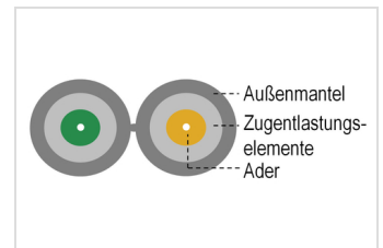
Duplexpatchkabel Querschnitt
