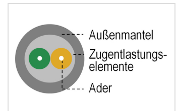
Duplexpatchkabel Jumperkabel Querschnitt
