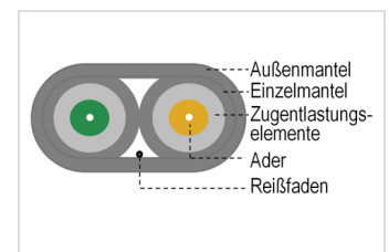
Duplexbreakoutkabel Querschnitt
