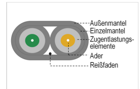
Duplexbreakoutkabel Querschnitt
