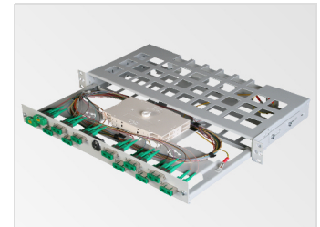
1 HE Spleißschublade, bestueckt
