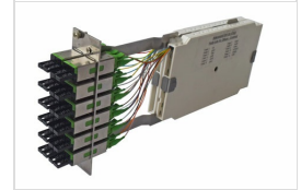
Compact Splice Module Twin E2000
