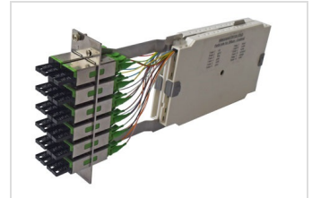
Compact Splice Module Twin E2000
